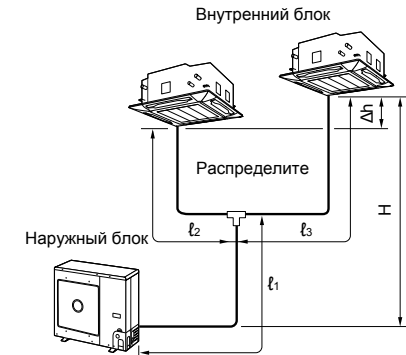
Рисунок одновременно сдвоенного трубопровода
