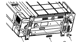
Водонепроницаемая резиновая крышка (5 шт.)
