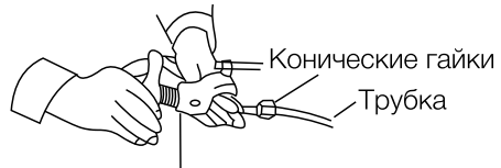
Развальцовочный инструмент
