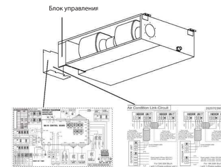
Монтажная схема
